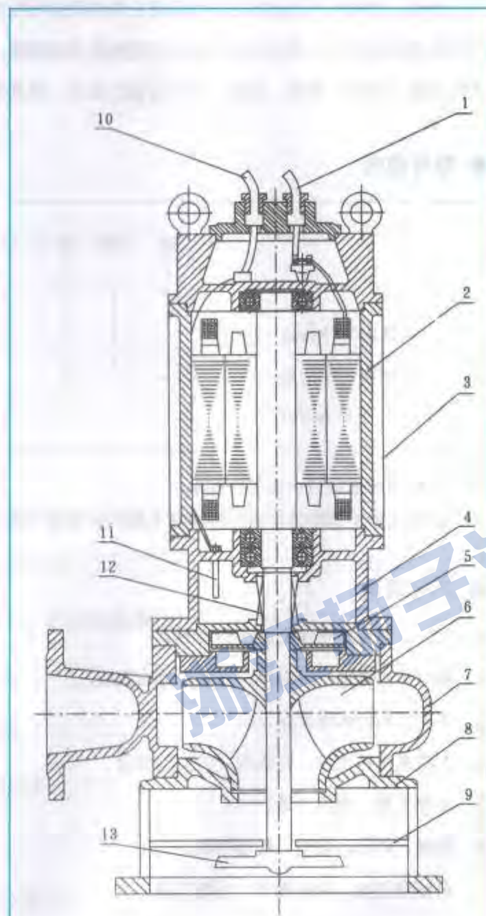
1—主电缆 2—机壳 3—内循环套 4—油箱 5—副叶轮 6—叶轮 7—泵体 8—底座 9—隔板 10—控制电缆 11—油水探头 12—机械密封 13—搅拌件
