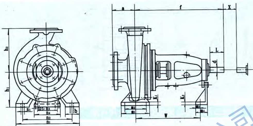
泵及泵脚座尺寸图
