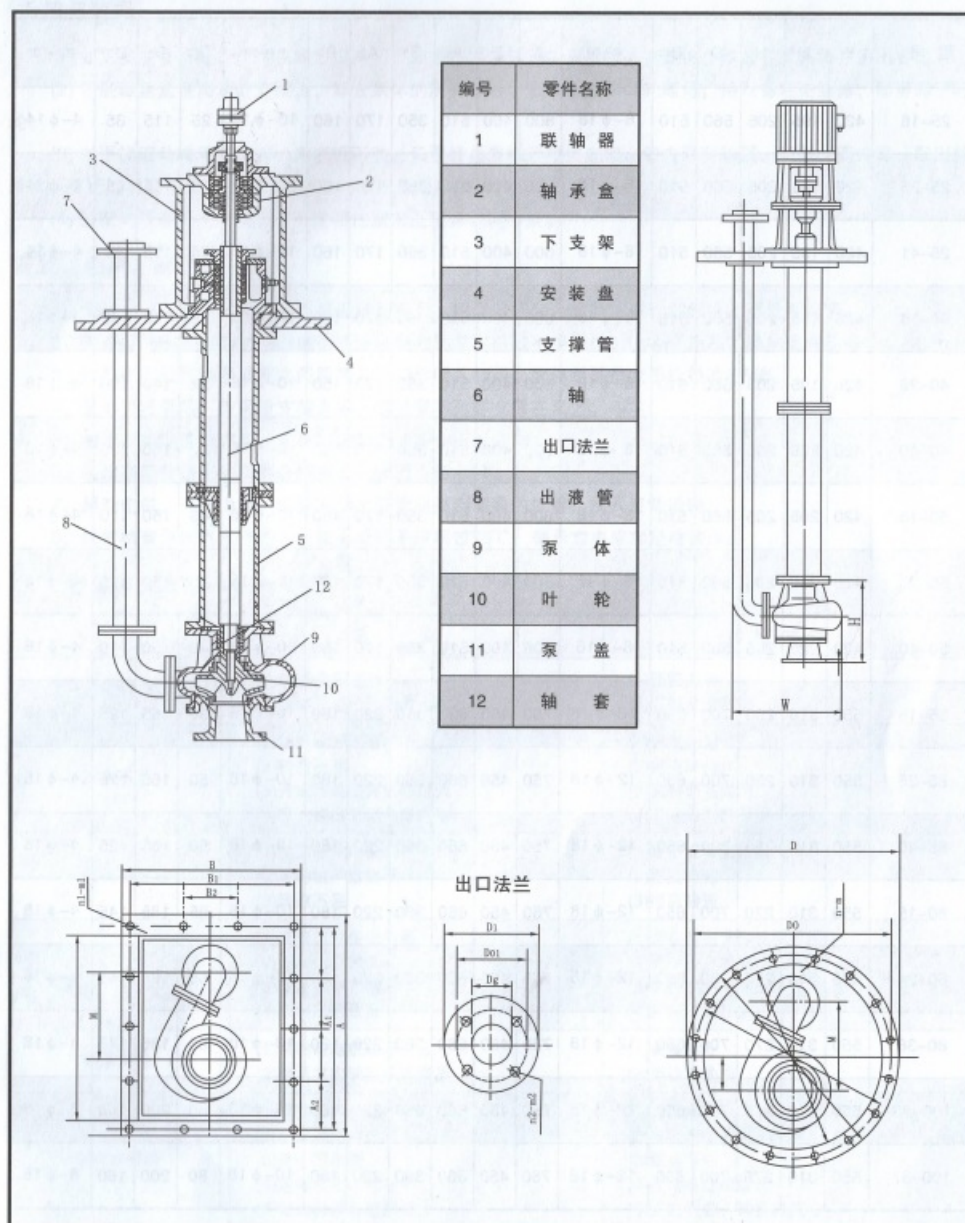
&lt;&lt;&lt; FY型液下泵结构图及安装尺寸图 &gt;&gt;&gt;
