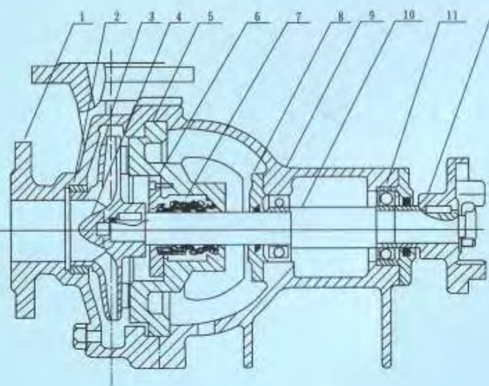
FB、AFB型结构图
