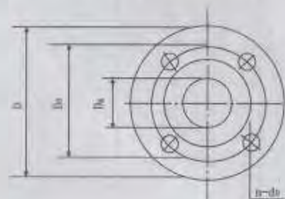
吸入吐出法兰
