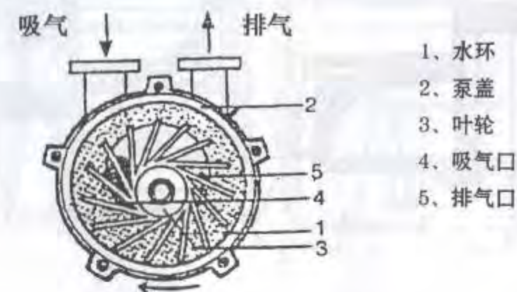
图1 水环真空泵及压缩机工作原理图
